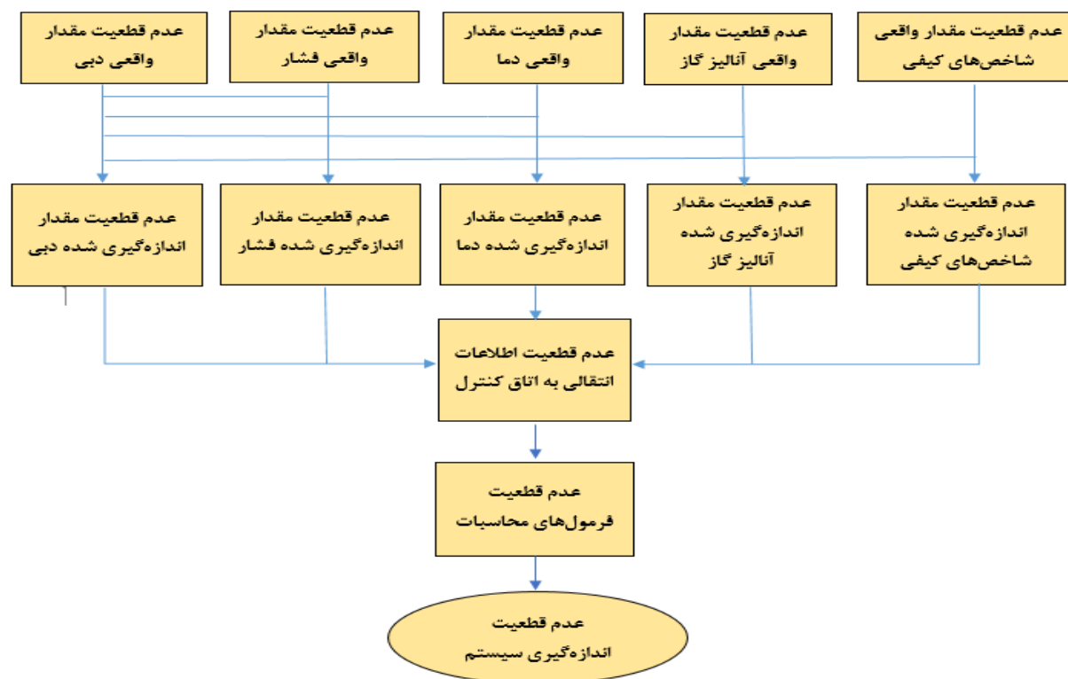
شکل ۲: فلوچارت زنجیره عدم قطعیت سیستم اندازه‌گیری گاز طبیعی
