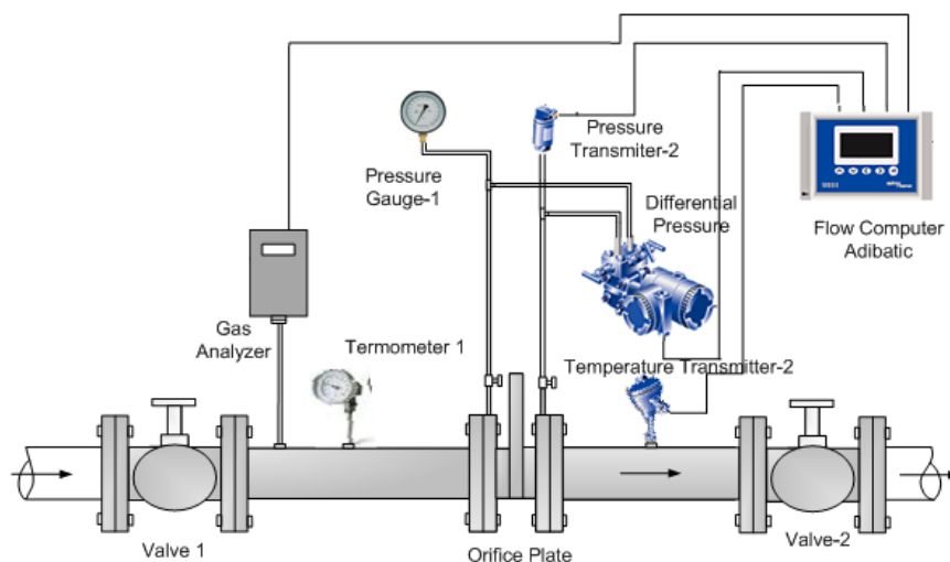
شکل ۱: یک ایستگاه اریفیزی به همراه متعلقات آن
