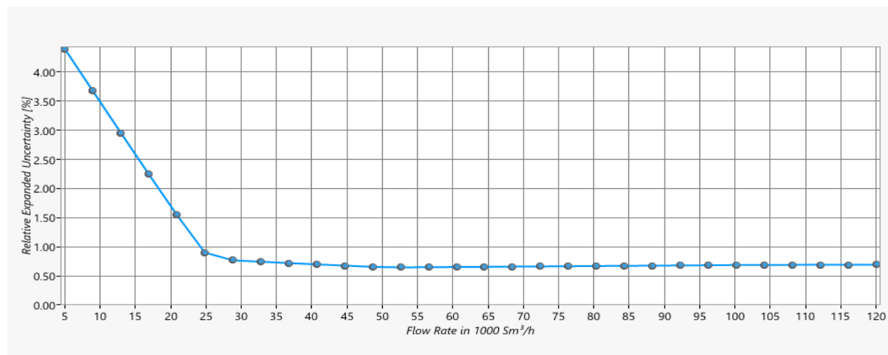
شکل ۶- تغییرات درصد عدم قطعیت بر حسب دبی گاز عبوری ایستگاه CGS ۱۲۰ هزار متر مکعبی نکا شرکت گاز استان مازندران
