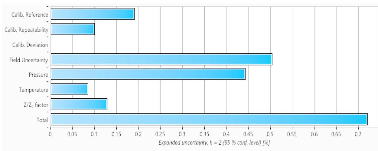
شکل ۵: عدم قطعیت پارامترهای موثر و همچنین عدم قطعیت ترکیبی ایستگاه CGS ۱۲۰ هزار متر مکعبی نکا شرکت گاز استان مازندران
