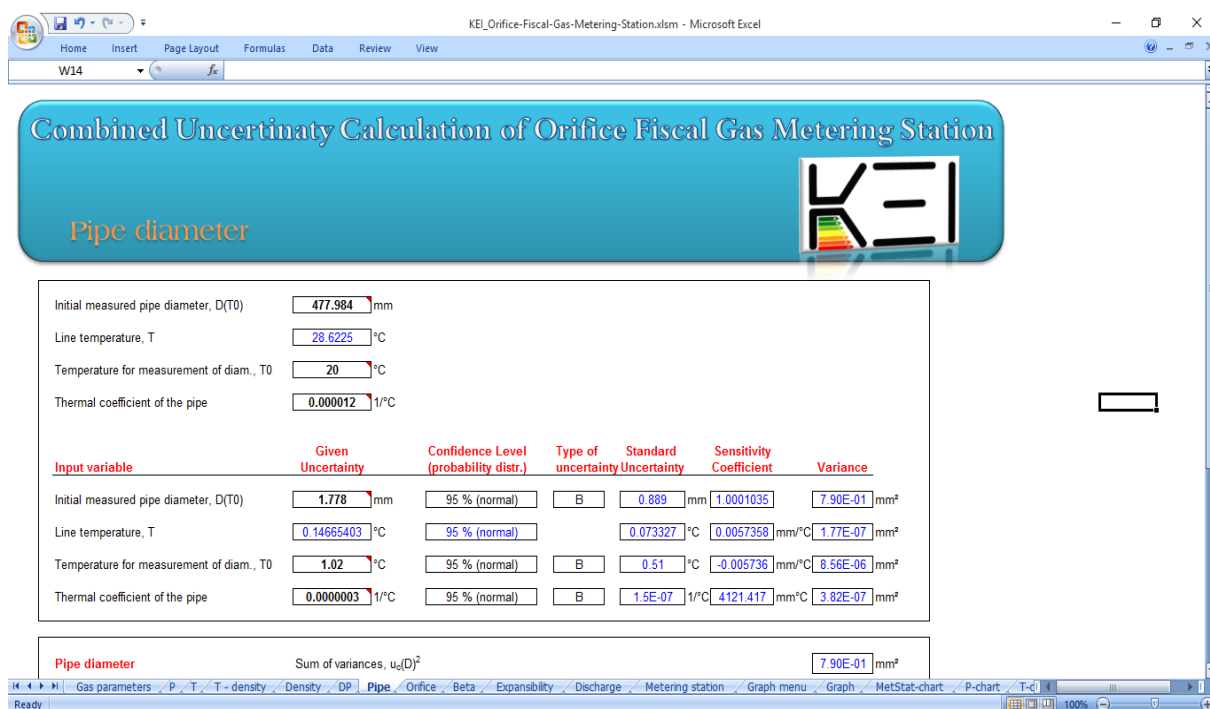
شکل ۴. تصویر فایل اکسل ایجاد شده جهت محاسبه عدم قطعیت ترکیبی گاز (زیربرگ مشخصات لوله)
