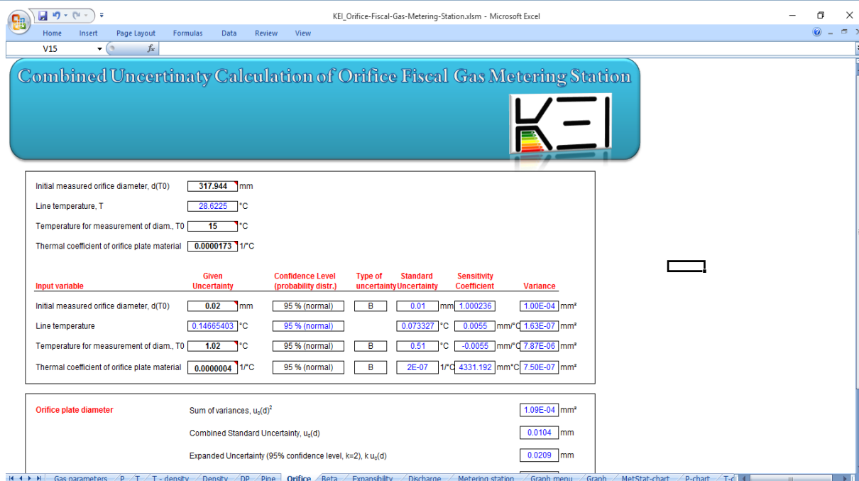
شکل ۳. تصویر فایل اکسل ایجاد شده جهت محاسبه عدم قطعیت ترکیبی گاز (زیربرگ مشخصات صفحه اریفیس)
